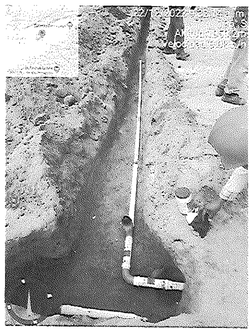
Supervisión instalación de red de tubería hidráulica de Ø 2" barrio portal de la victoria
